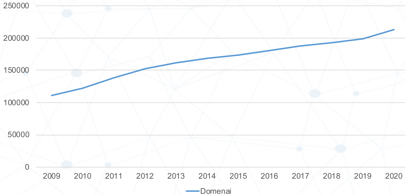
Registruotų .lt domenų skaičius
